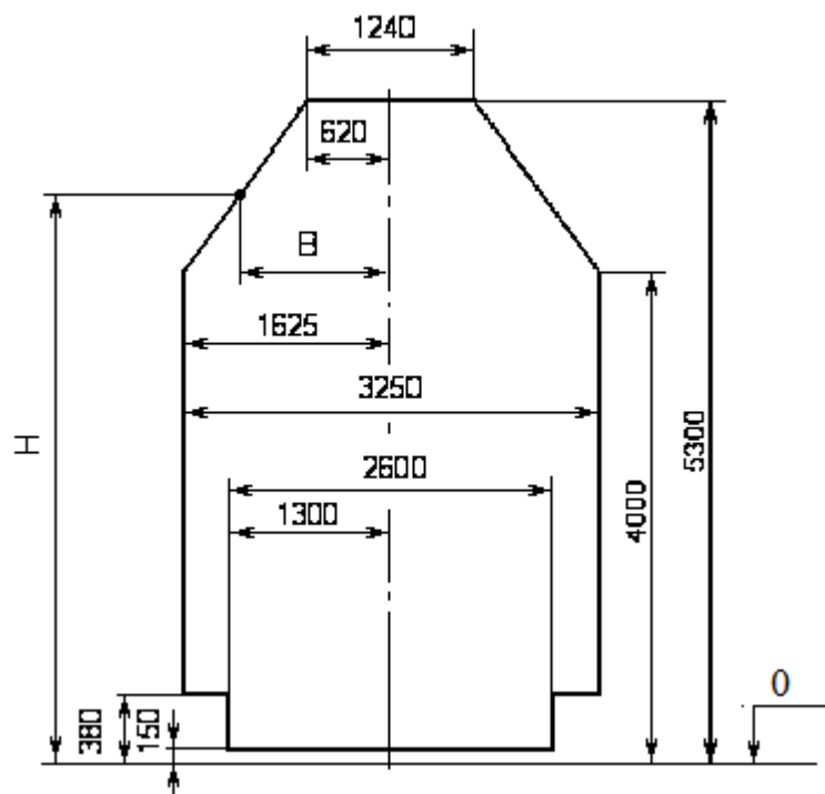
Рисунок 1 – Очертание основного габарита погрузки на железных дорогах России Значения расстояния В от вертикальной плоскости, проходящей через ось железнодорожного пути, до точек очертания габаритов на высоте Н от уровня головок рельсов (далее УГР) – «0», приведены в таблице 2.
