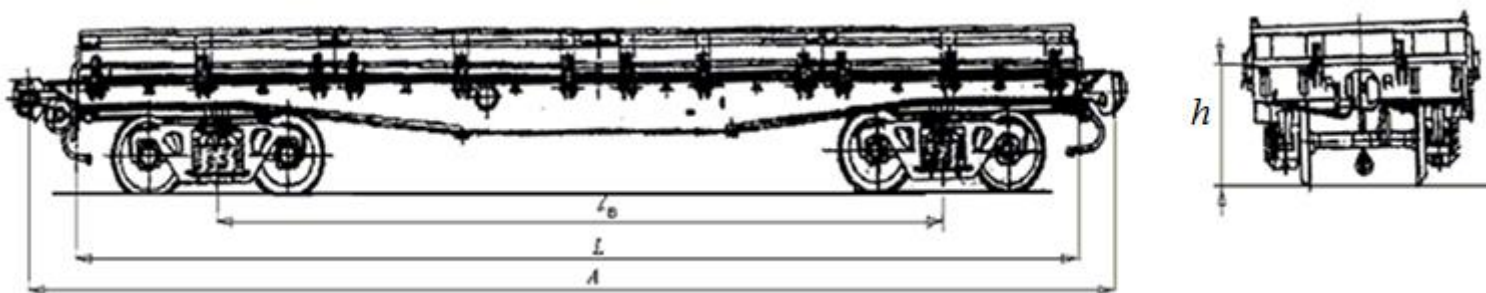
Рисунок 6 – Платформы
