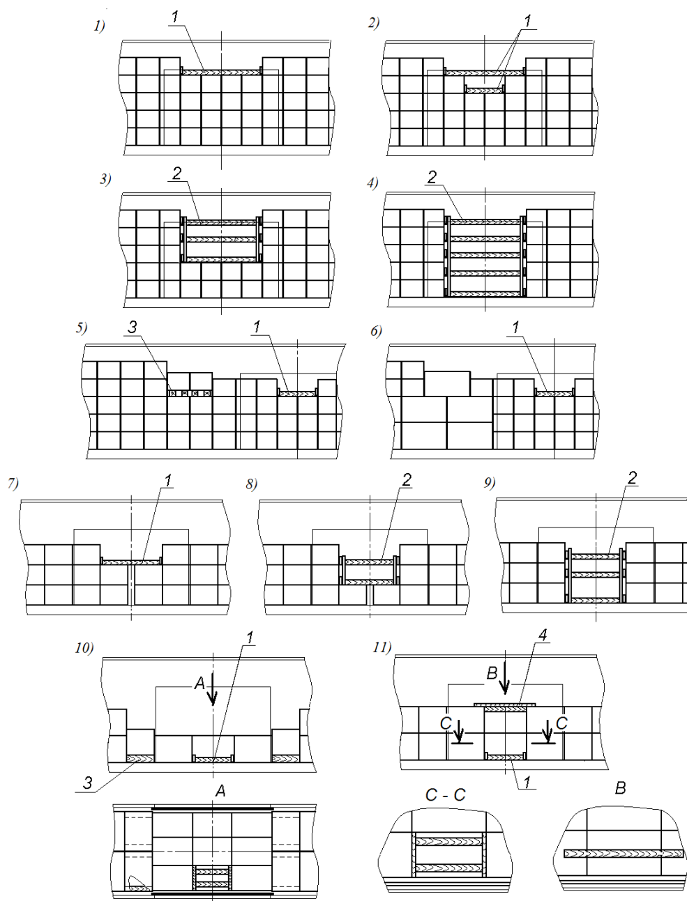
Рисунок 14 – Примеры крепления ящиков, пакетов в продольном направлении 1 – распорная рама; 2 – распорная конструкция; 3 – подкладка; 4 – накладка-распорка
