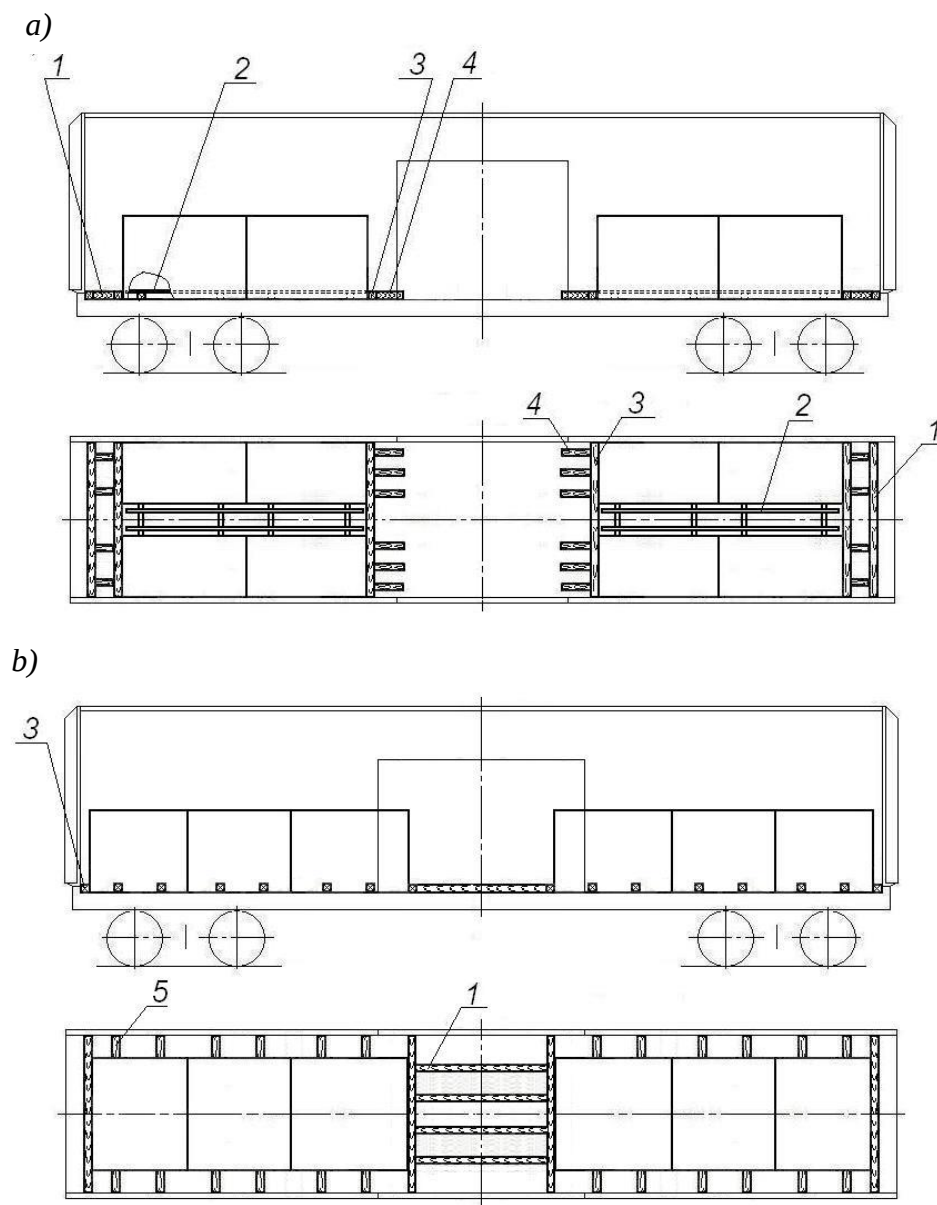
Рисунок 32 – Крепление отдельных мест груза в вагонах с деревянным и деревометаллическим полом 1, 2 – распорная рама; 3, 4 – упорный брусок; 5 – распорный брусок
