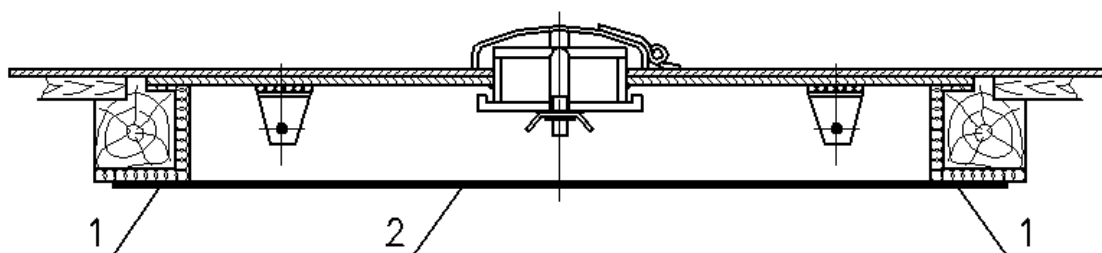
Рисунок 6 – Заделка печной разделки бумагой
