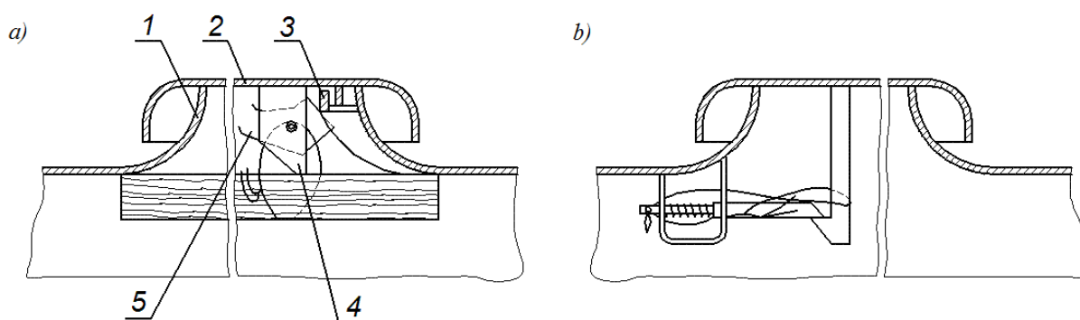
Рисунок 4 – Увязка верхних загрузочных люков
