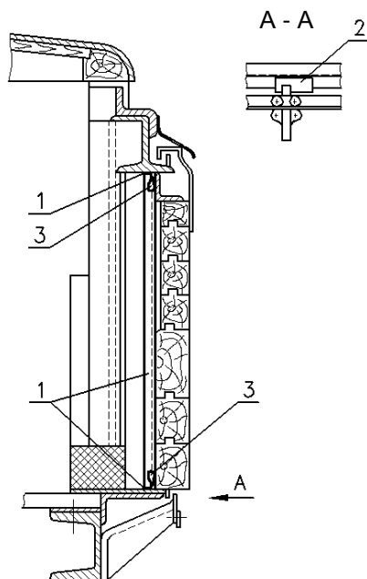
Рисунок 7 – Заделка зазоров двери вагона, используемой для погрузки, бумагой
