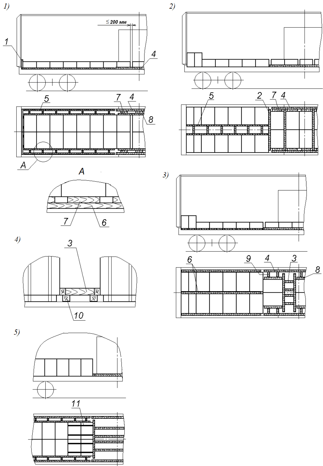
Рисунок 24 – Примеры размещения и крепления пакетов цветных металлов 1 – торцевой щит; 2, 8 – упорные бруски; 3, 5 – распорные рамы; 4 – брусок ограждения дверного проема; 6, 7, 9 – распорные бруски; 10 – подкладка; 11 – увязка
