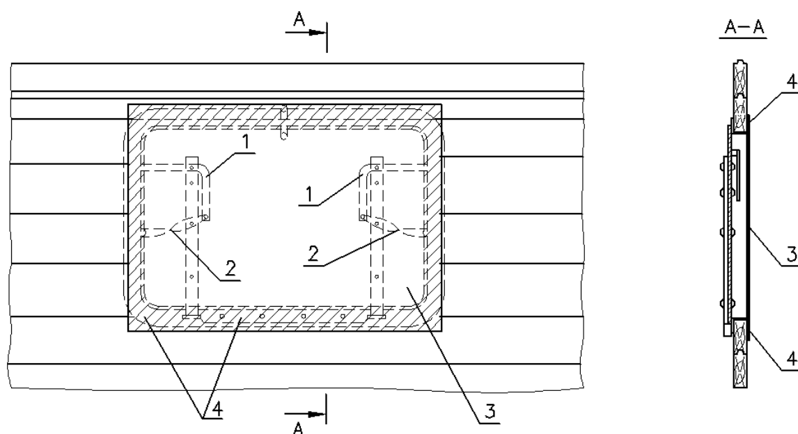
Рисунок 5 – Заделка бокового люка бумагой 1 – закидка люка; 2 – проволоочная увязка; 3 – бумага; 4 – место приклеивания бумаги (заштриховано)
