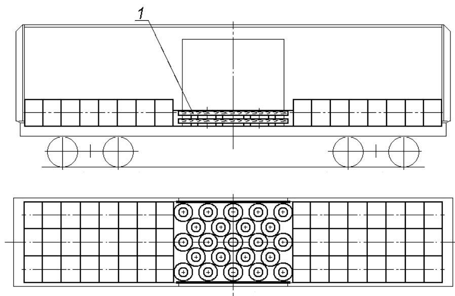
Рисунок 27 – Пример комбинированного размещения бунтов 1 – ограждение дверного проема
