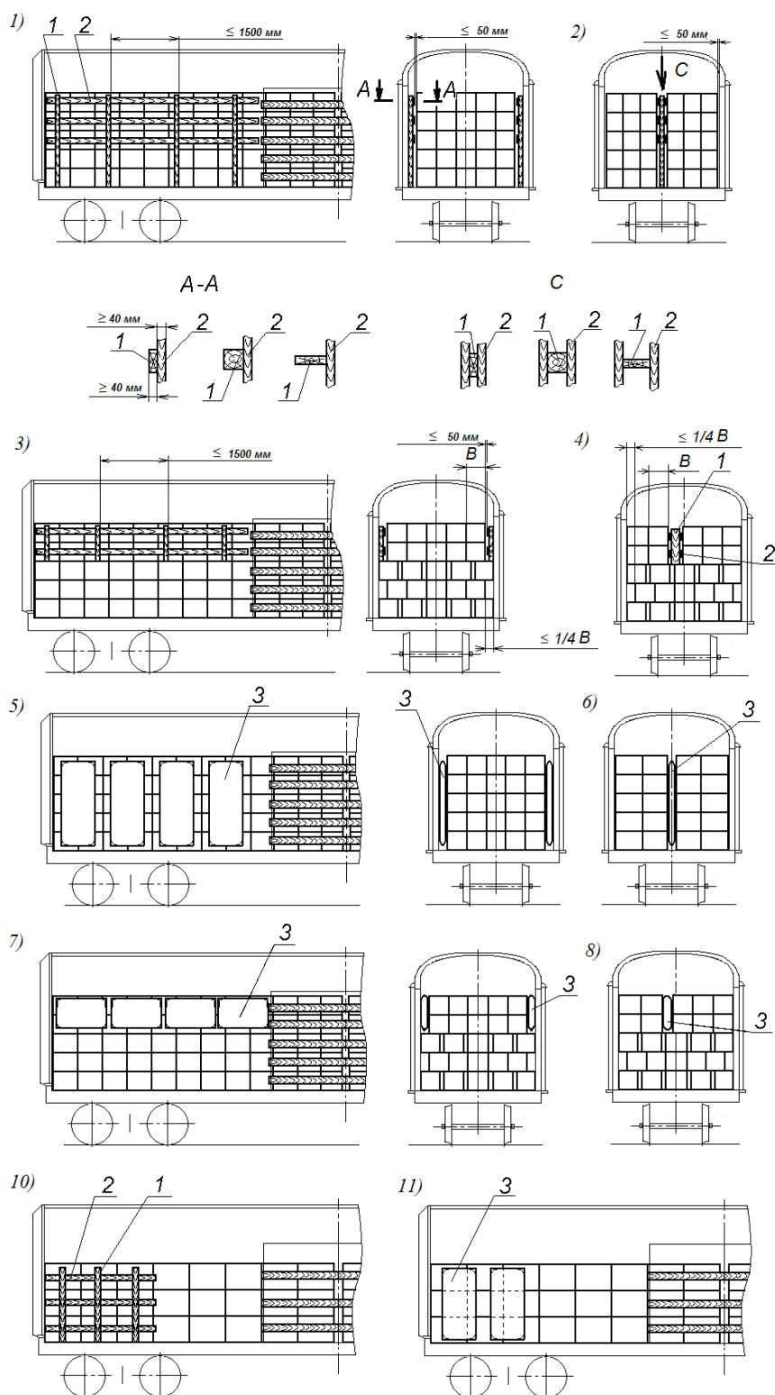
Рисунок 17 – Примеры крепления ящиков, пакетов в поперечном направлении:
