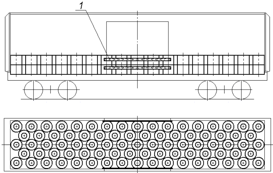
Рисунок 25 – Пример размещения бунтов на торец 1 – ограждение дверного проема
