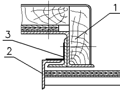
Рисунок 8 – Заделка зазоров между вертикальными стойками дверного проема и створкой двери 1 – стойка дверного проёма; 2 – створка двери; 3 – стеклоткань
