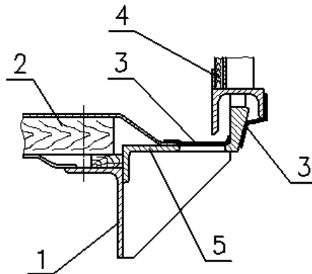
Рисунок 9 – Заделка зазора в месте соединения пола со створкой двери и порогом дверного проема 1 – продольная балка рамы вагона; 2 – пол; 3 – стеклоткань; 4 – створка двери; 5 – порог дверного проема
