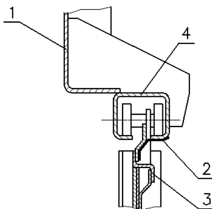
Рисунок 10 – Заделка зазора в месте соединения створки двери с направляющим рельсом
