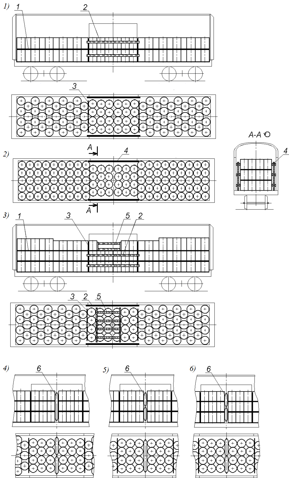
Рисунок 18– Примеры размещения и крепления грузов в бочках, барабанах 1 – прокладочный материал; 2 – доска ограждения дверей; 3 – щит; 4 – распорный щит; 5 – распорная конструкция; 6 – пневмооболочка
