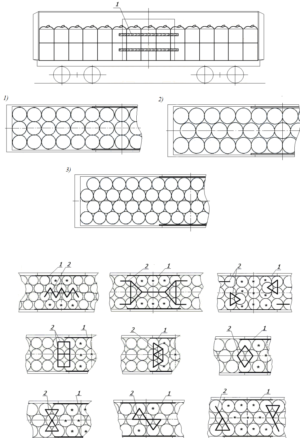
Рисунок 29 – Примеры размещения и увязки мягких контейнеров
