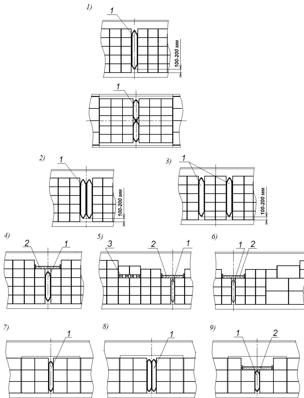
Рисунок 16 – Примеры крепления ящиков, пакетов в продольном направлении с использованием пневмооболочек
