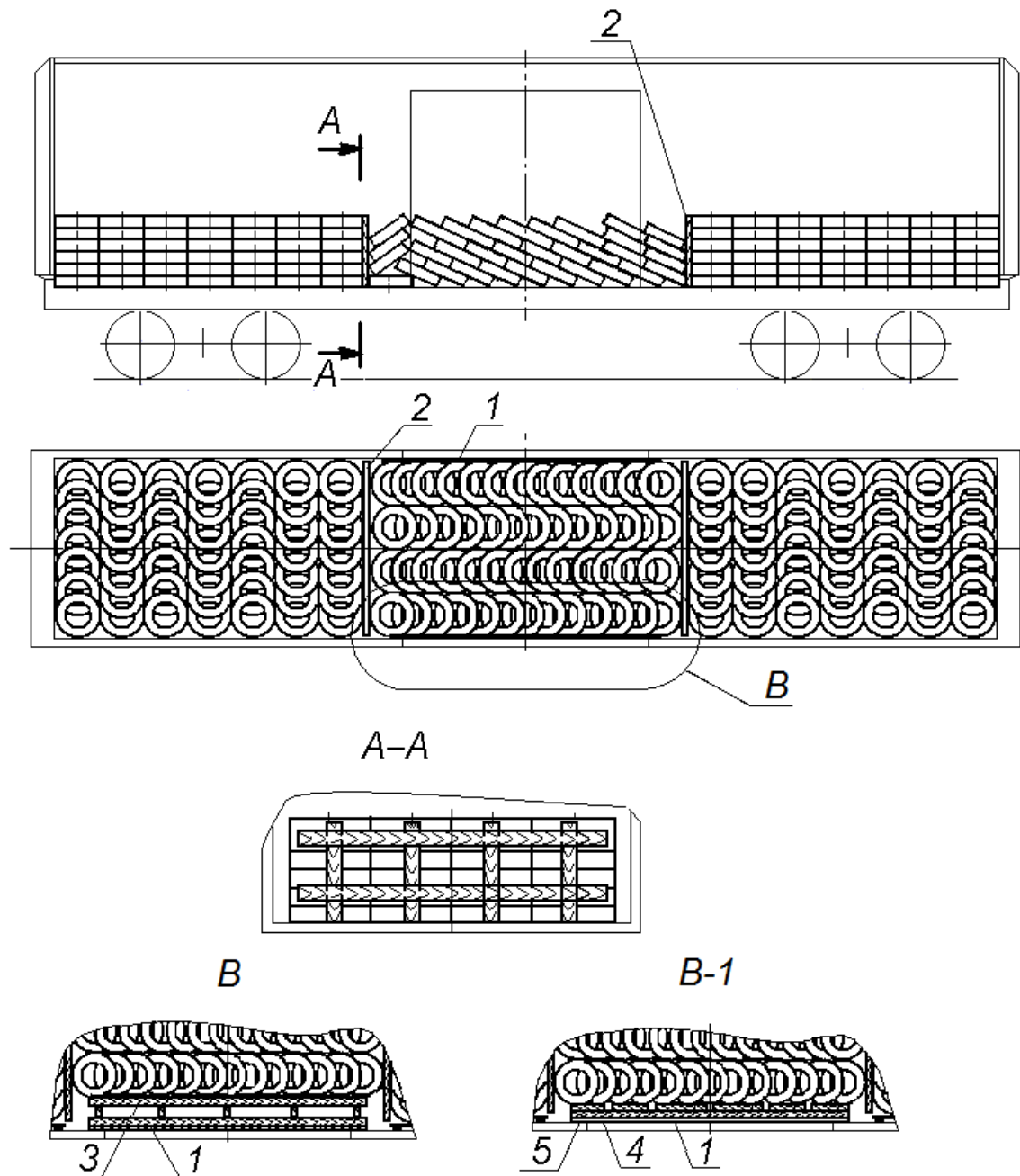
Рисунок 26 – Пример размещения бунтов в наклонном положении 1 – ограждение дверного проема; 2 – распорный щит; 3 – распорная рама; 4 – упорный брусок; 5 – распорный брусок
