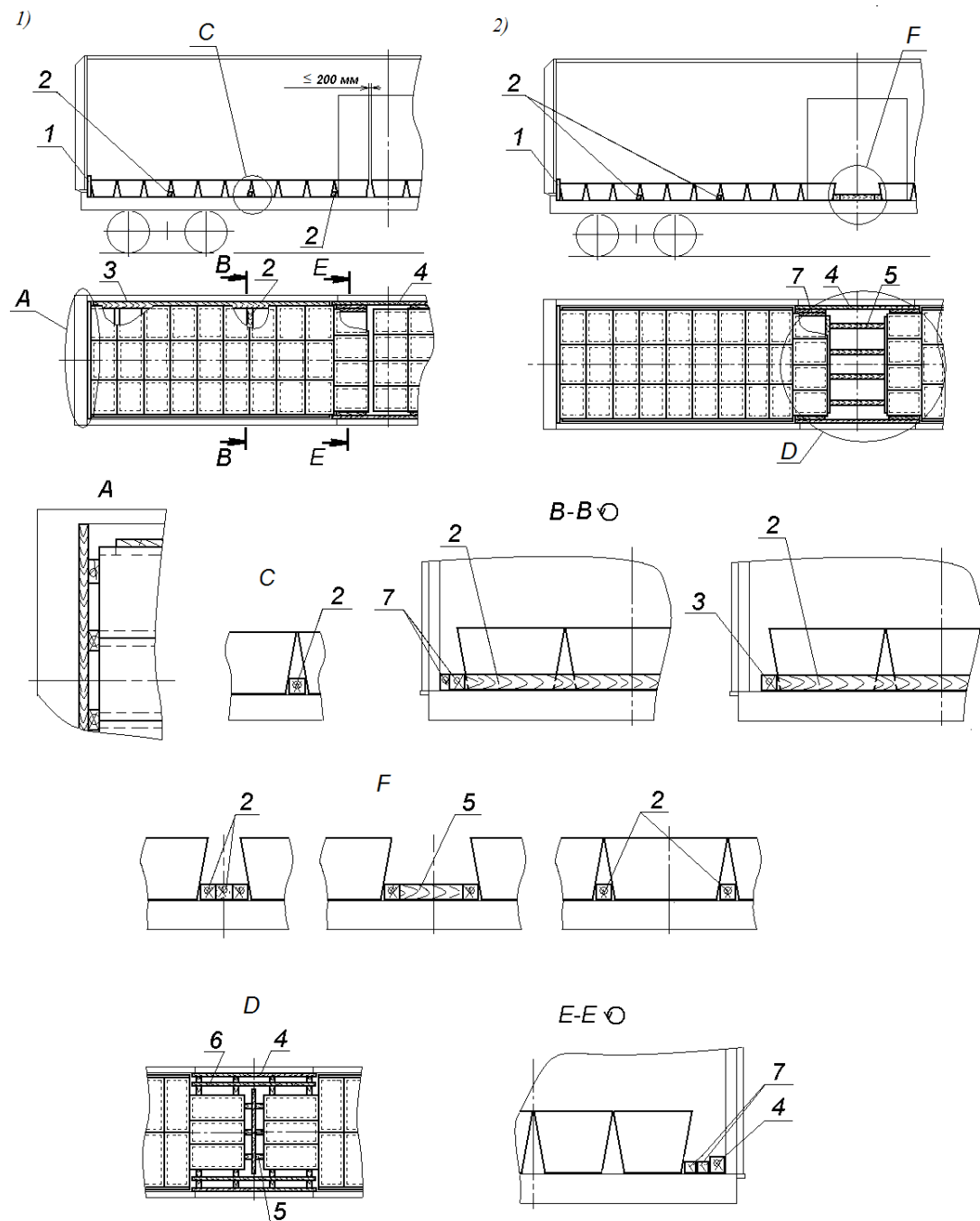
Рисунок 23 – Примеры размещения и крепления слитков 1 – торцевой щит; 2, 3 – упорные бруски; 4 – брусок ограждения дверного проема; 5, 6 – распорные рамы; 7 – распорные бруски
