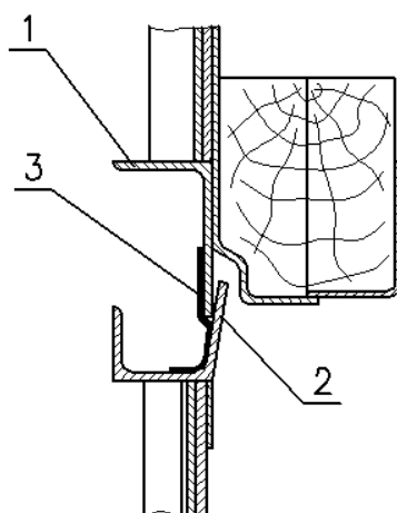
Рисунок 11 – Заделка зазора между створками двери
