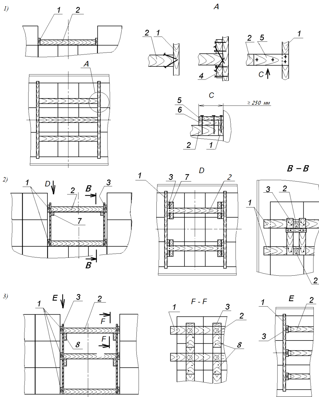
Рисунок 15 – Распорная рама, распорная конструкция 1 – упорная доска; 2 – распорный брусок; 3 – стойка; 4 – брусок; 5 – накладка; 6 – доска; 7, 8 – опорные бруски; А- варианты крепления упорных досок и распорных брусков.
