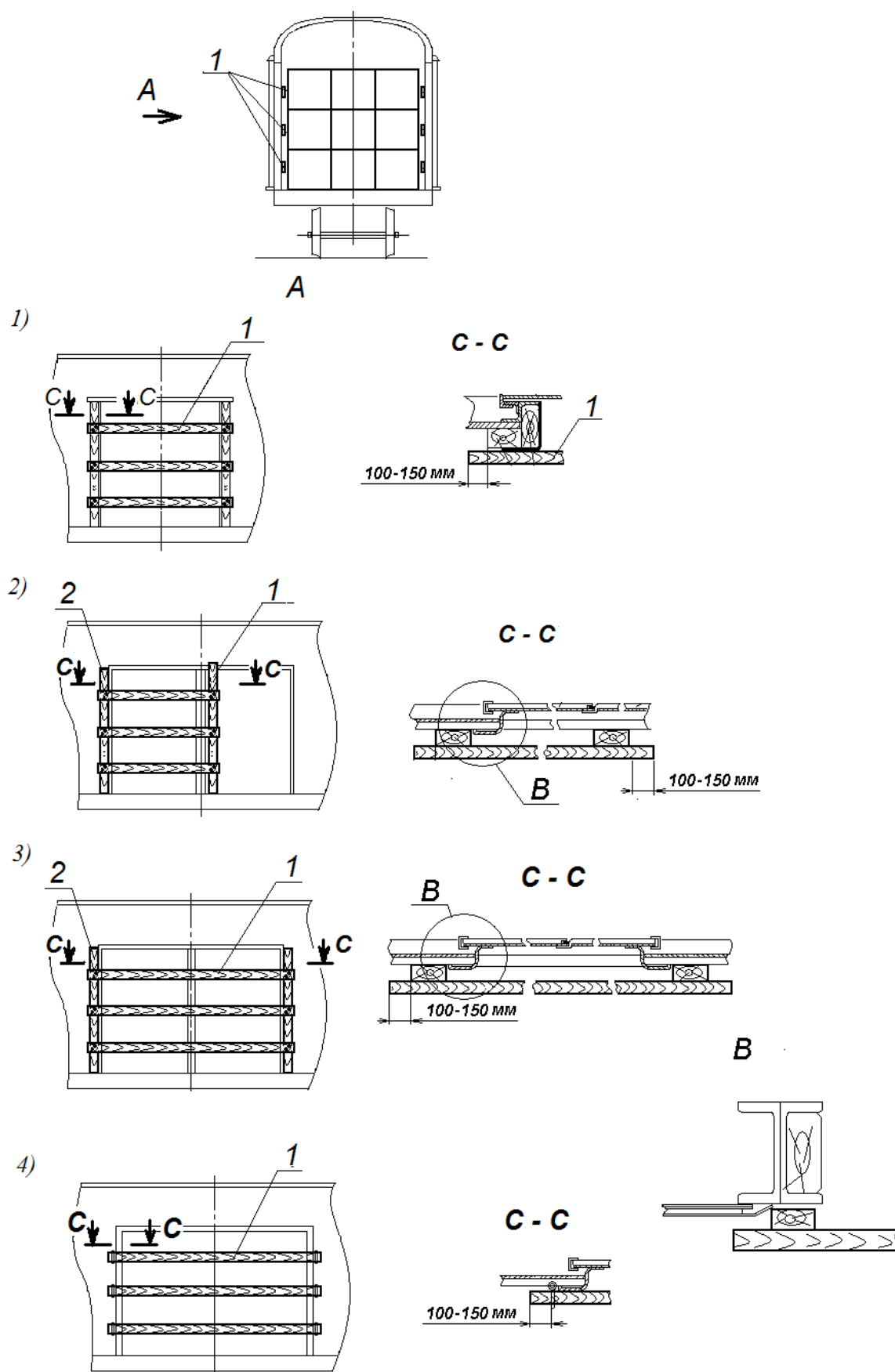
Рисунок 3 – Варианты ограждения дверей 1 – горизонтальная доска; 2 – стойка
