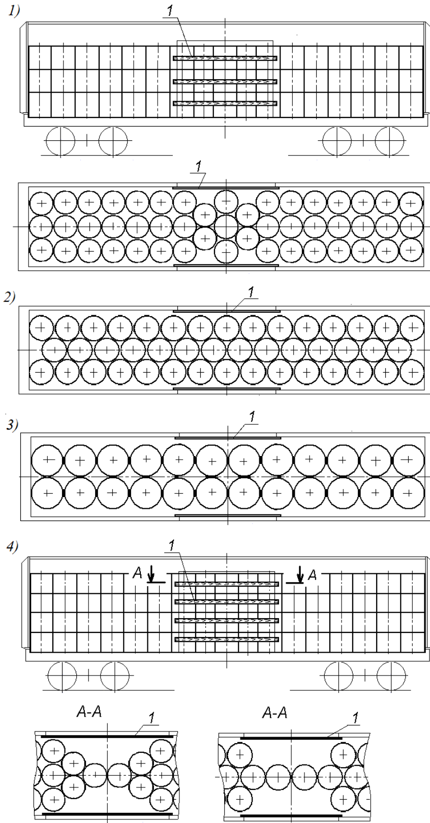
Рисунок 19 – Примеры размещения рулонов бумаги и картона 1 – доска ограждения дверей
