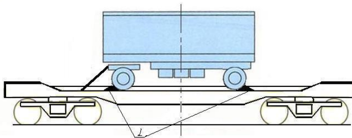
Рисунок 15 – Размещение и крепление прицепа 1 – колесный упор
