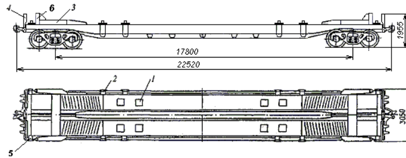
Рисунок 2 – Платформа модели 13-4095
