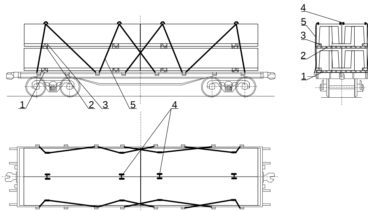
Рисунок 22 – Размещение и крепление лотков марок Л10 – Л13
