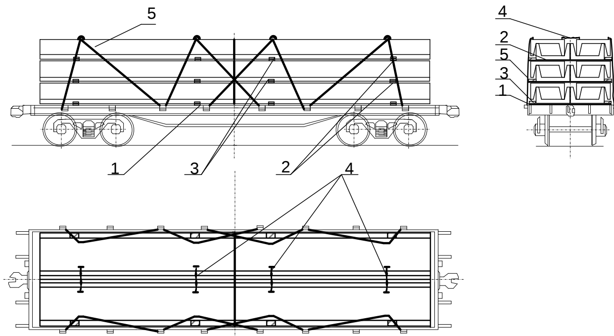
Рисунок 21 – Размещение и крепление лотков марок Л6 – Л9
