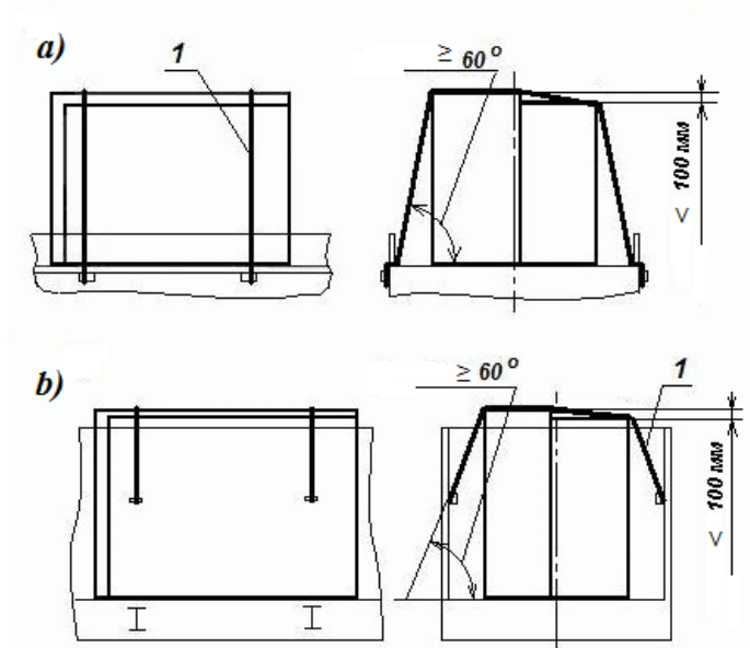
Рисунок 16 – Крепление от опрокидывания группы ящиков обвязками: (средства крепления от смещений условно не показаны)
