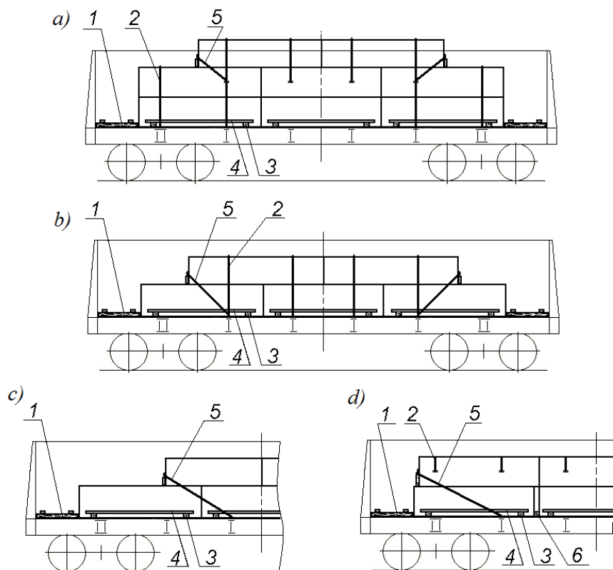
Рисунок 20 – Принципиальные схемы крепления групп ящиков в неполных по длине ярусах:
