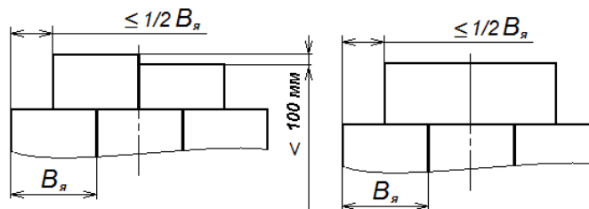
Рисунок 19 – Размещение ящиков в верхнем ярусе штабеля
