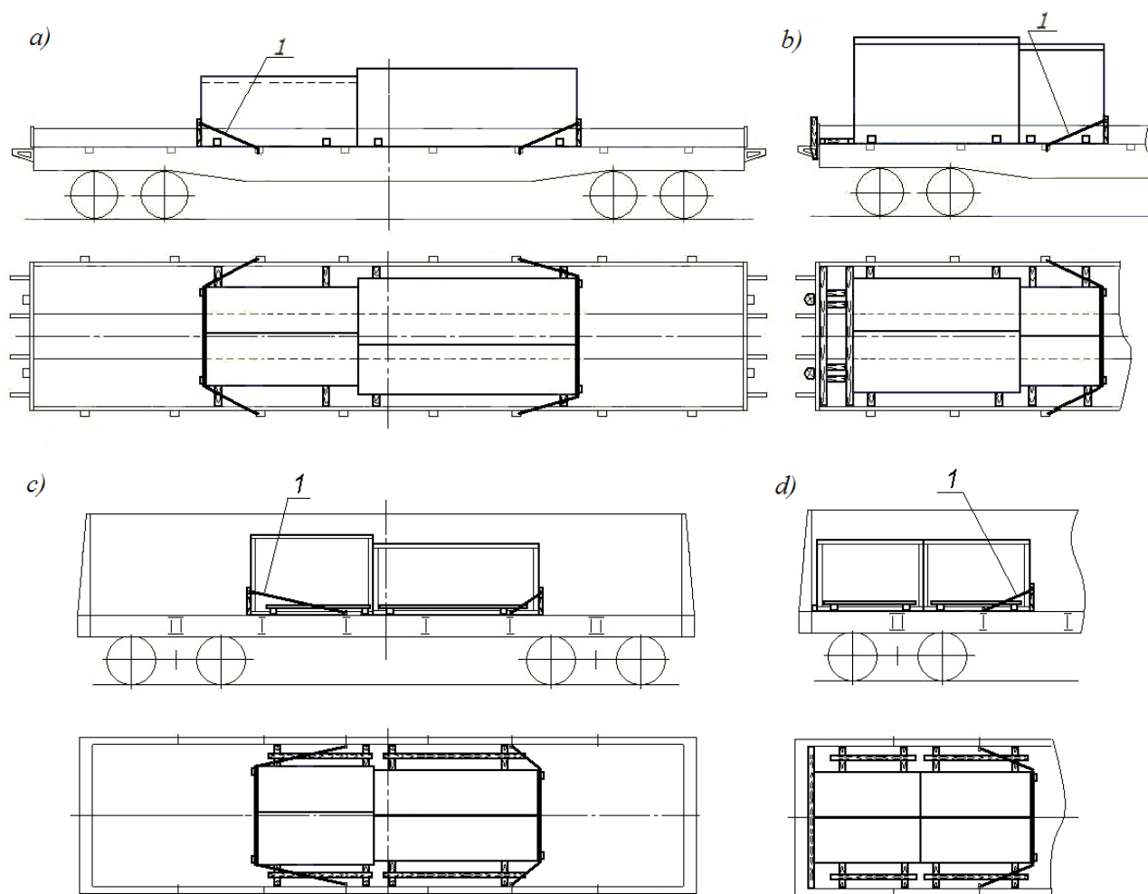
Рисунок 15 – Принципиальные схемы крепления группы ящиков наклонными обвязками: а, б – на платформе; с, д – в полувагоне
