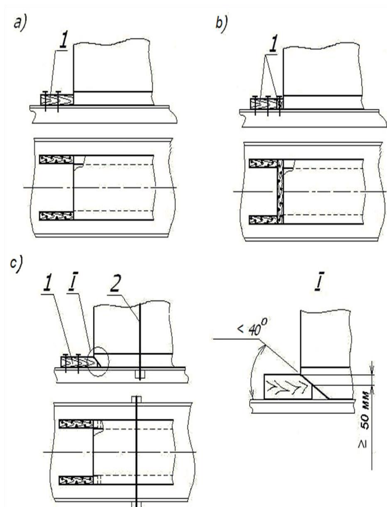
Рисунок 8 – Примеры крепления груза на салазках в продольном направлении брусками:
