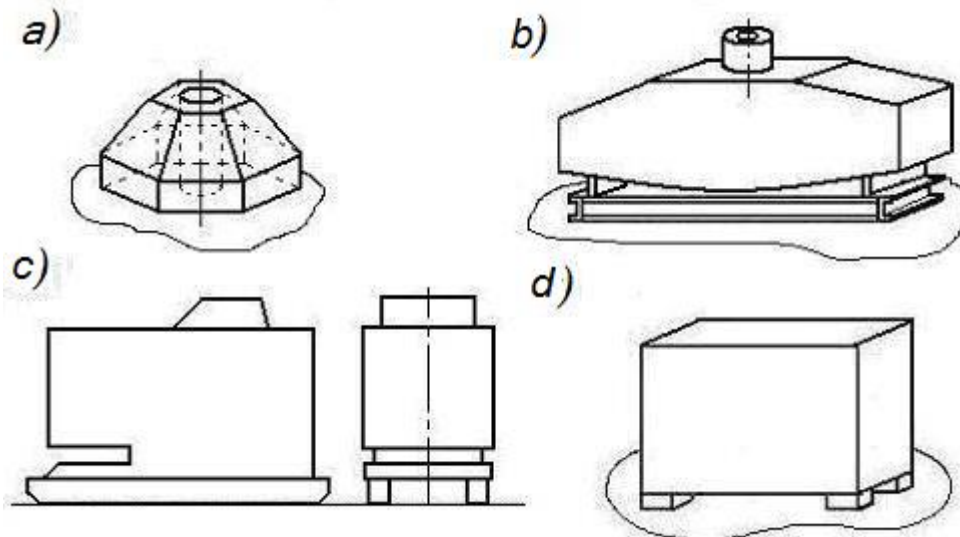
Рисунок 1 – Примеры грузов с плоскими опорами: а – груз с плоской опорной поверхностью; б – груз на опорной раме; с – груз на салазках; д – груз на отдельных опорах
