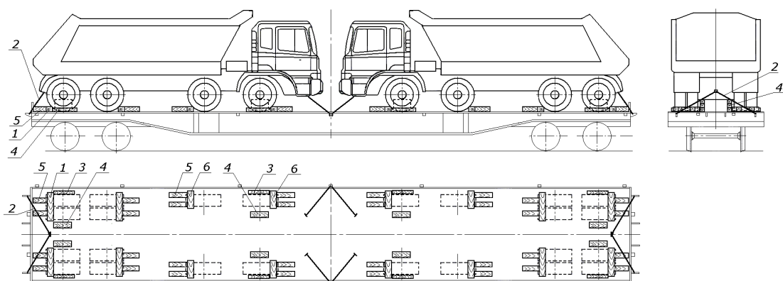
Рисунок 4 1 – упорный брусок от продольного смещения; 2 – растяжка; 3 – упорный брусок от поперечного смещения; 4 – подставка
