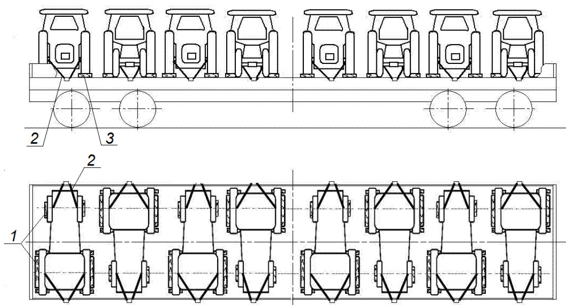
Рисунок 21 – Размещение и крепление техники на обрешеченных колесах поперек платформы
