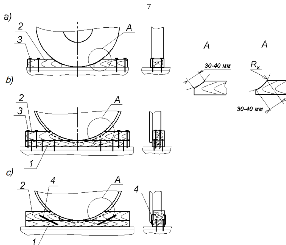
Рисунок 17 – Подклинивание металлических колес техники при нагрузке от колеса до 2,0 т включительно
