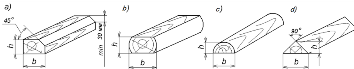
Рисунок 7 – Варианты исполнения упорных брусков для подклинивания обрешиненных колес из:
