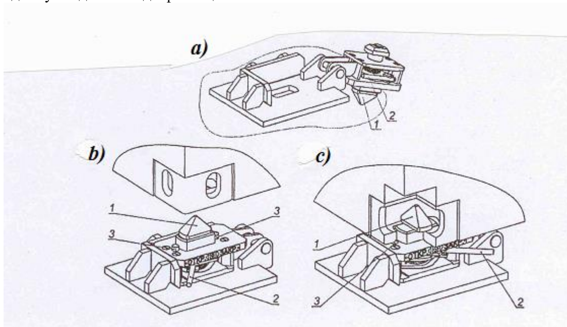
Рисунок 51 - Упор для крепления контейнеров а - нерабочее положение упора;
