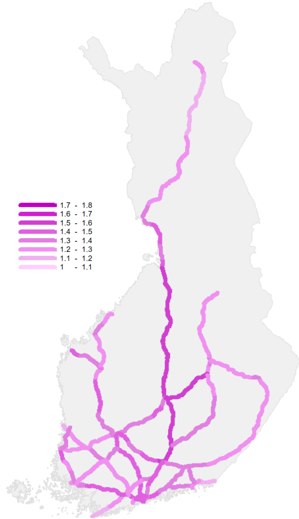
Pääteiden vilkkaiden yhteysvälien kasvukertoimet kevyille ajoneuvoille 2021-2050
