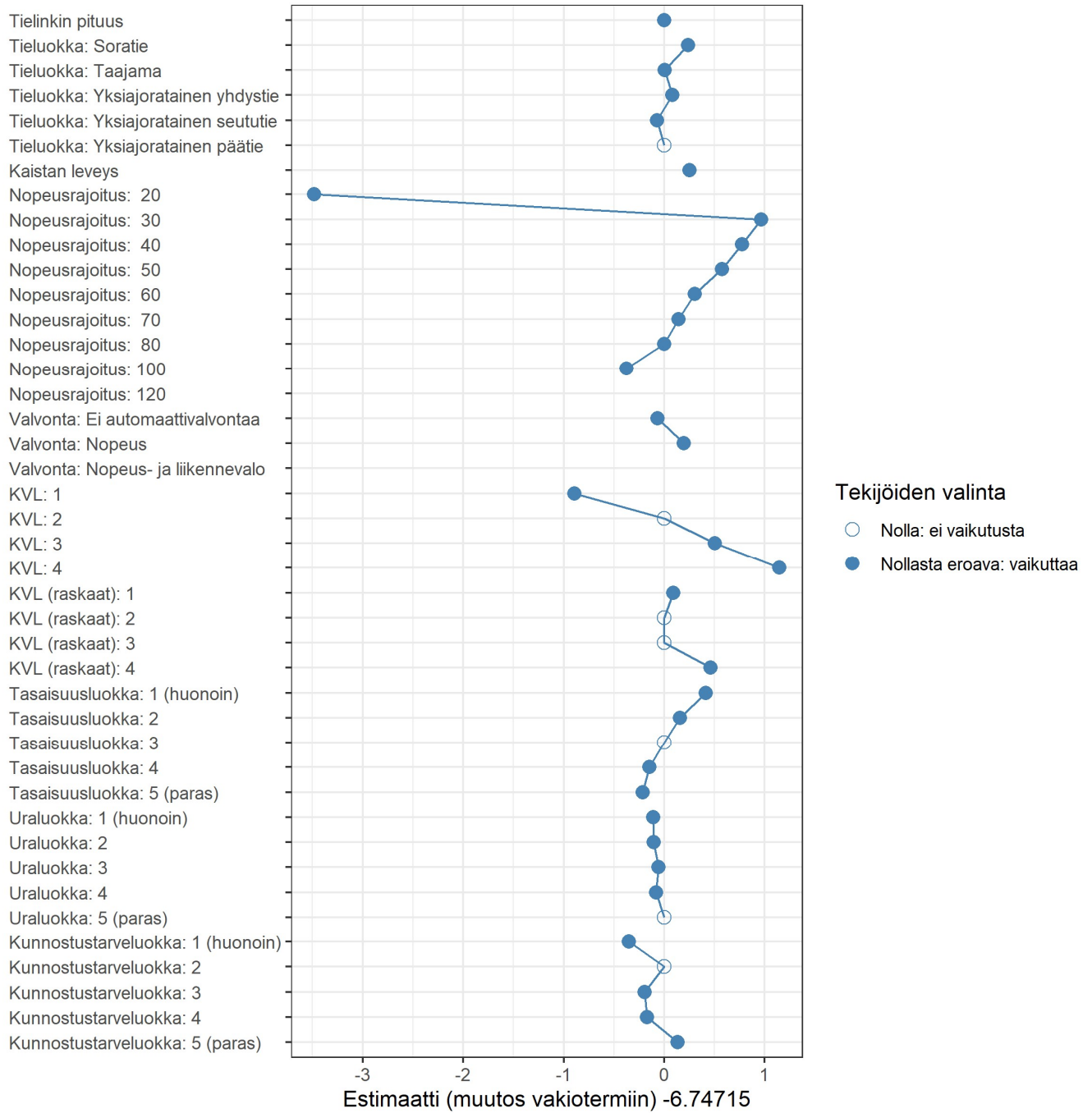
Kuva 3. Onnettomuusmallin kertoimet.
