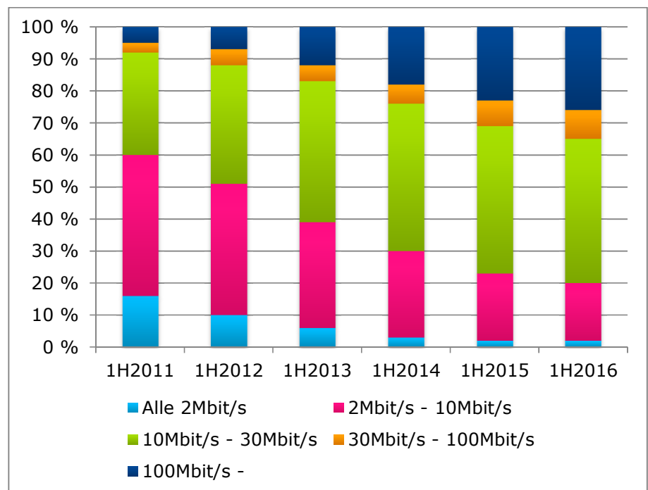
Kuvio 3. Kiinteän verkon laajakaistaliittymien nopeusluokkien jakauma.
