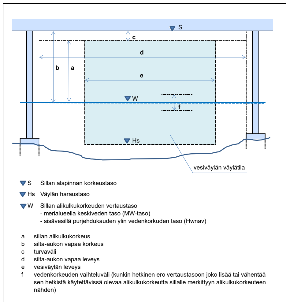
Kuva 1. Yleisen kulkuväylän ylittävän vesistösillan silta-aukkoon liittyvät käsitteet
