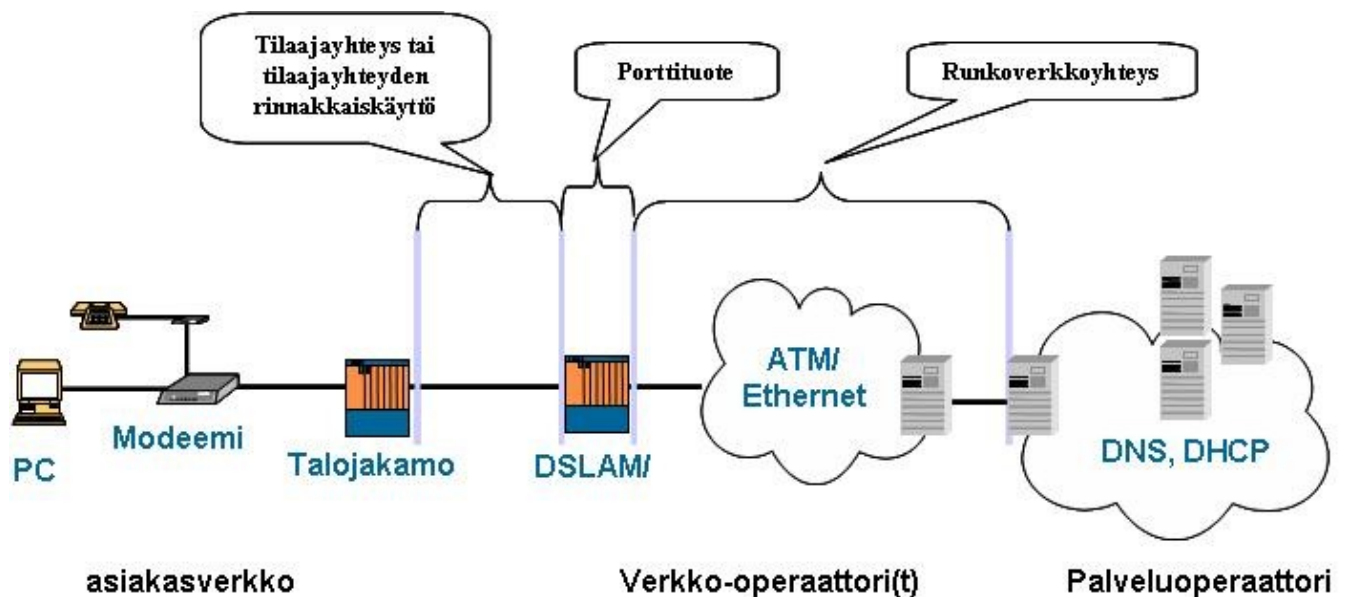
Kuva 1: Laajakaistayhteystuotteet
